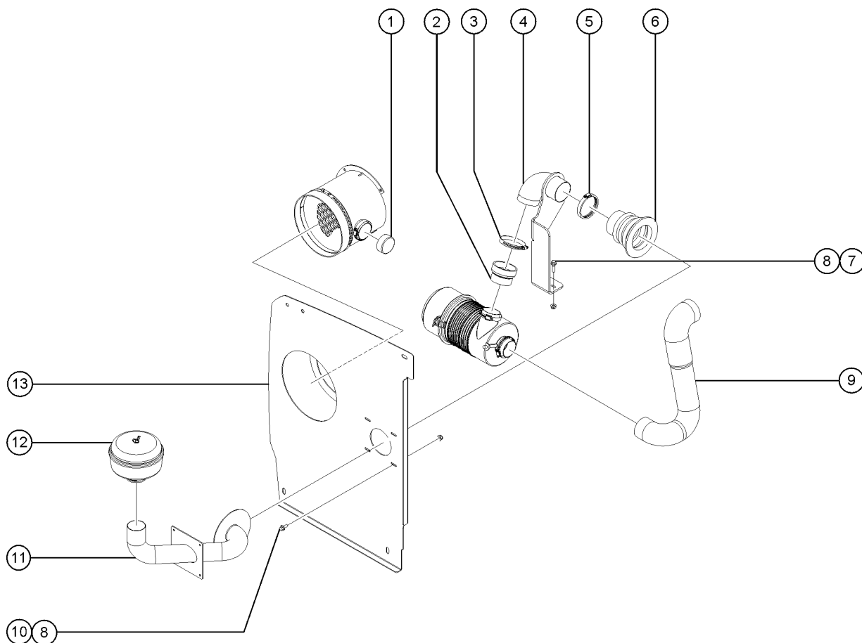
Deutz D2011L03i
